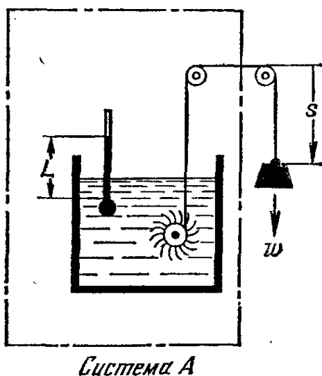
Рис. 5.6. Система A состоит из сосуда с водой, термометра и колеса с лопастями. Падающий груз совершает работу над этой системой.
