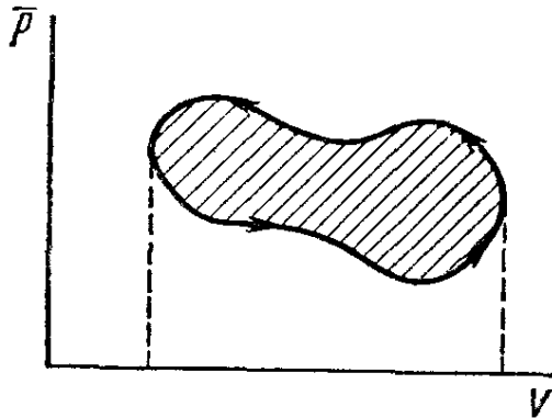
Рис. 5.17. Циклический процесс
