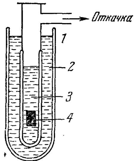
Рис. 5.4. Типичное устройство из двух сосудов Дьюара для работы вблизи 1^\circ\text{K} . Дьюар, наполненный жидким гелием, помещен в другой дьюар, наполненный жидким азотом. Такое устройство уменьшает проникновение тепла в жидкий гелий. 1 — окружающая среда при 295^\circ\text{K} , 2 — жидкий азот при 77^\circ\text{K} , 3 — жидкий гелий при 4,2^\circ\text{K} , 4 — охлажденный образец при низкой температуре.
