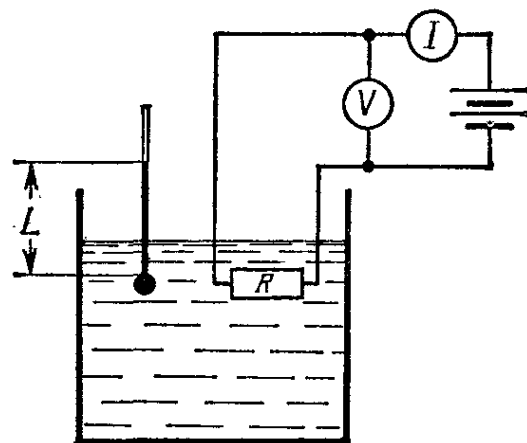
Рис. 1.32. Два различных термометра находятся в тепловом контакте с системой, состоящей из сосуда, наполненного жидкостью. Один термометр ртутный и его термическим параметром является длина столбика ртути в стеклянном капилляре термометра. Другой термометр представляет собой электрическое сопротивление R , сделанное из платиновой проволоки или из угля. Его термическим параметром является электрическое сопротивление R (определяемое током I , текущим через сопротивление, и напряжением V на нем).
