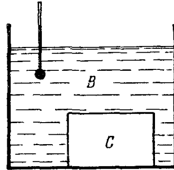
Рис. 5.12. Количество тепла, поглощенное куском меди C , измеряется по количеству тепла, отданному известной системой B , состоящей из сосуда с водой и термометра.
