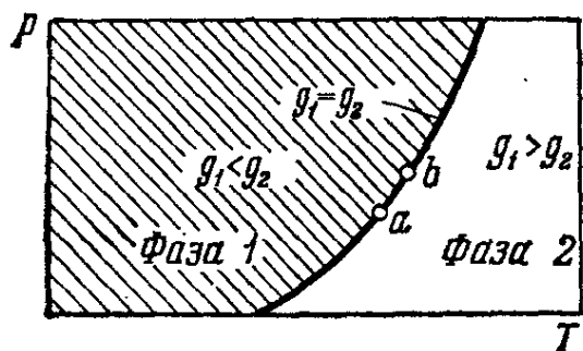
Рис. 7.10. Кривая зависимости давления p от температуры T , разделяющая область, где каждая из двух фаз в отдельности может находиться в равновесии. Вдоль кривой возможно совместное равновесное состояние обеих фаз.
