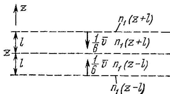
Рис. 8.9. Перенос меченых молекул через плоскость.
