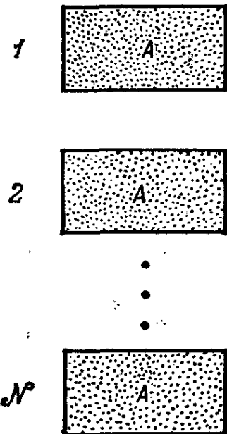
Рис. 2.2. Статистическое описание системы A , представляющей собой газ, заключенный в ящик. На рисунке схематически показан статистический ансамбль из \mathcal{N} систем, подобных рассматриваемой системе A .
