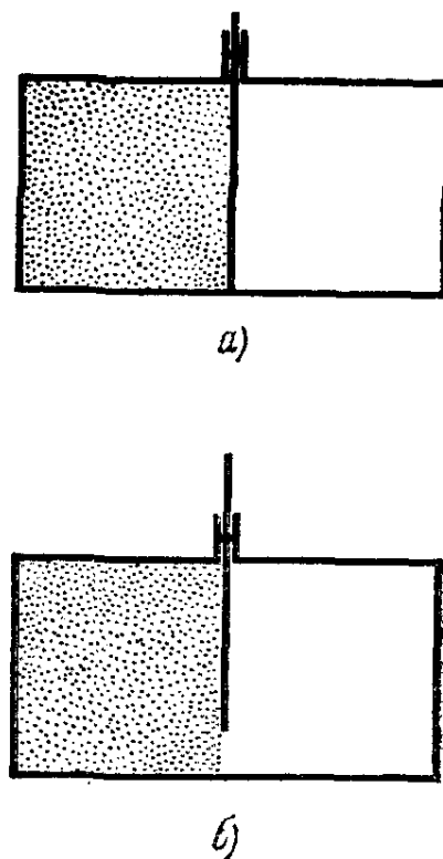
Рис. 1.13. Перегородка неожиданно поднята, но не до конца.
