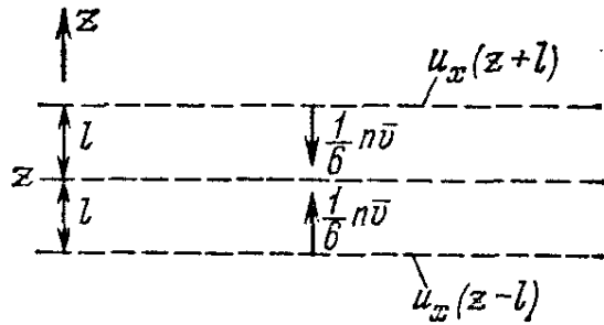
Рис. 8.5. Молекулы, пересекающие плоскость, осуществляют перенос импульса.
