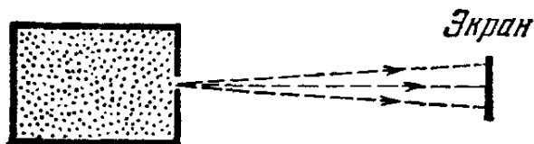
Рис. 6.15. Эффузионный пучок падает на экран.
