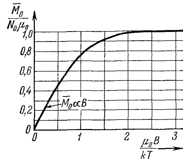
Рис. 4.10. Зависимость намагниченности \bar{M}_0 от магнитного поля B и температуры T в случае слабо взаимодействующего атома со спином 1/2 и магнитным моментом \mu_0 .
