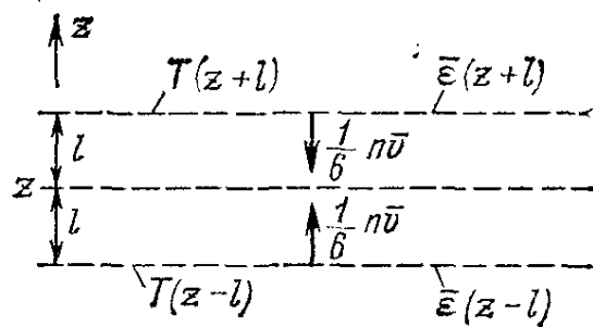
Рис. 8.7. Молекулы, пересекающие плоскость, переносят энергию.
