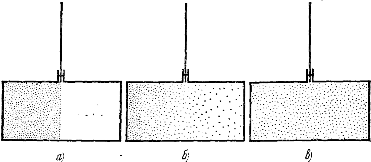
Рис. 1.11. а) Ящик из рис. 1.10 сразу же после того, как была убрана перегородка, б) через небольшой промежуток времени и в) после того, как прошло достаточно много времени. Кинограмма, рассматриваемая в обратном направлении, будет показывать обратный порядок в), б), а).
