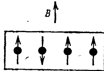
Рис. 2.5. Система из N спинов, равных 1/2 , в частном случае N=4 . Каждая стрелка показывает направление магнитного момента спина. Внешнее магнитное поле обозначено стрелкой \mathbf{B} .
