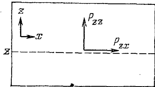
Рис. 8.3. Плоскость z = \text{const} в жидкости. Находящаяся ниже этой плоскости жидкость действует с силой P_z на жидкость над плоскостью.
