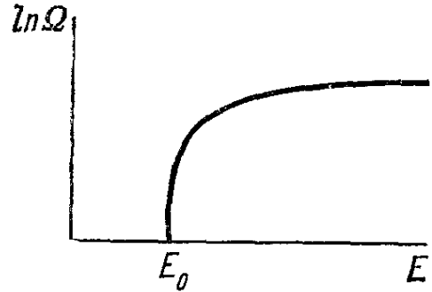
Рис. 4.5. Характер зависимости \ln \Omega от энергии E . Наклон кривой дает абсолютный температурный параметр \beta .
