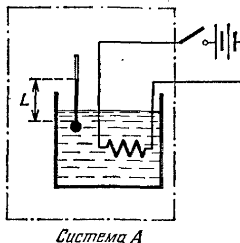
Рис. 5.7. Система A состоит из сосуда с водой, термометра и электрического сопротивления. Работа над этой системой совершается батареей
