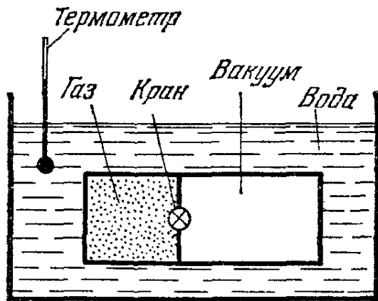
Рис. 5.19. Прибор для изучения свободного расширения газа.
