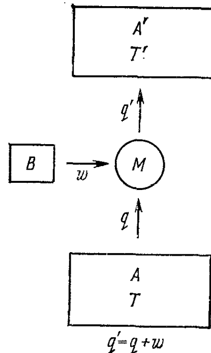
Рис. 7.15. Схема работы холодильника.
