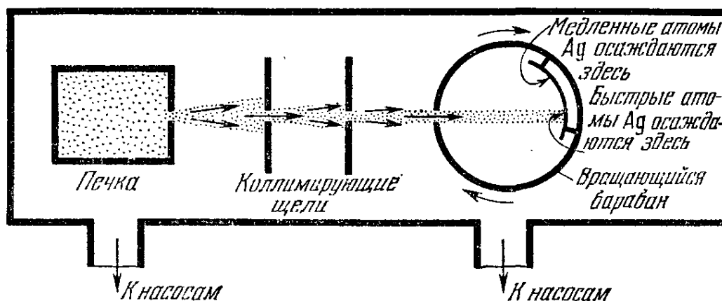
Рис. 6.10. Схема прибора с молекулярным пучком для изучения распределения скоростей атомов серебра (Ag). Ударившись о внутреннюю поверхность цилиндра, атомы остаются на ней.
