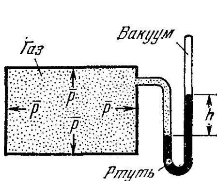
Рис. 1.33. Среднее давление газа \bar{p} измеряется при помощи манометра, состоящего из U-образной трубки, наполненной ртутью. В трубке устанавливается такая высота h столбика ртути, чтобы давление, оказываемое этим столбиком, уравновешивалось давлением газа.
