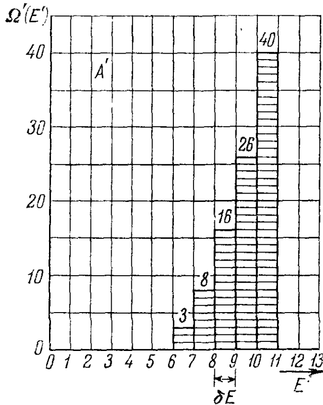
Рис. 4.1. На графиках показано (для частного случая двух очень малых систем A и A' ) числа состояний \Omega(E) и \Omega'(E') , доступных системам A и A' , в зависимости от энергии систем E и E' соответственно. Энергии измерены в произвольных единицах.
