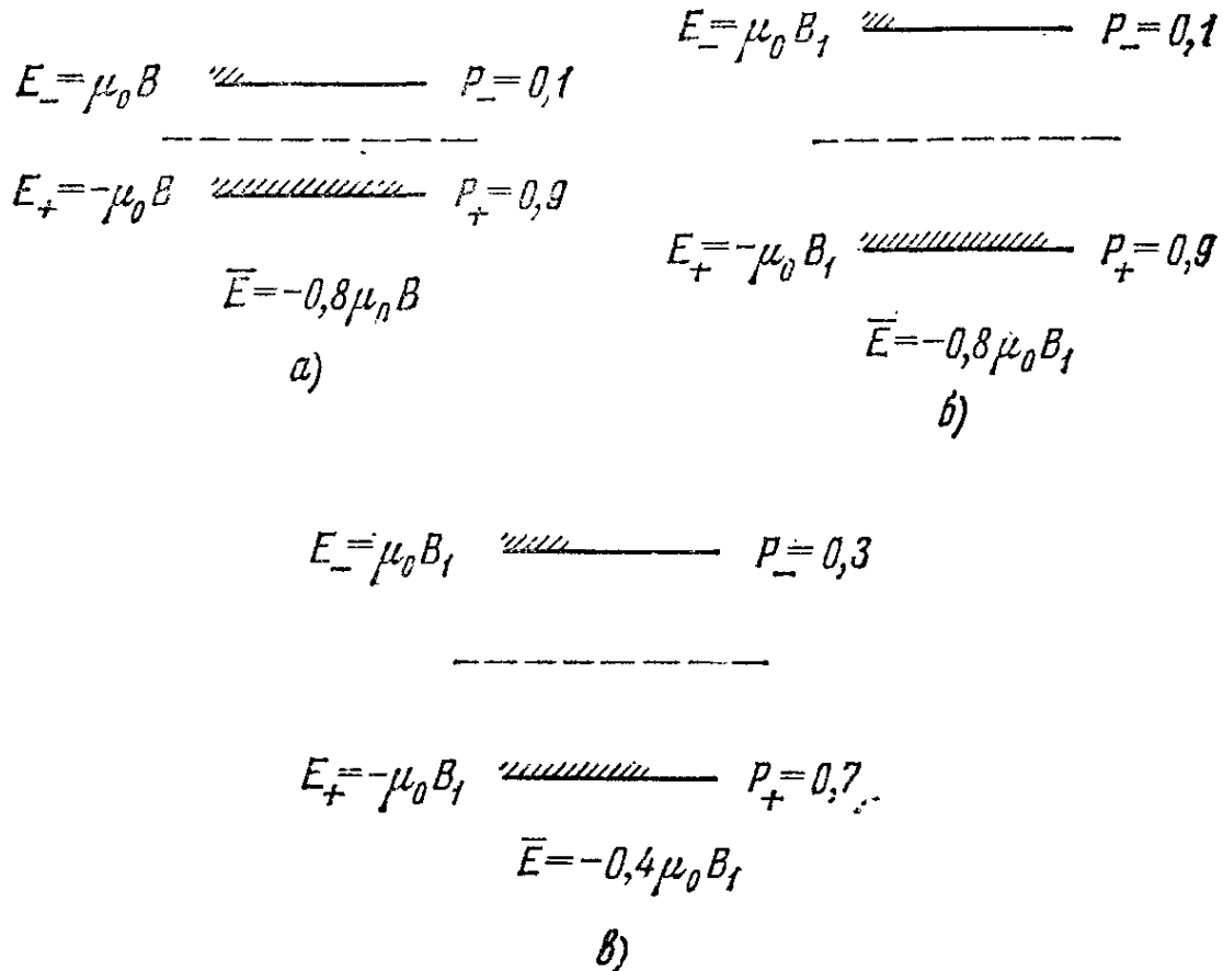
Рис. 3.13. Влияние адиабатического взаимодействия на очень простую систему A , состоящую из спина 1/2 с магнитным моментом \mu_0 , помещенную в магнитное поле B . Начальное положение и обозначения те же, что и на рис. 3.12, но спин адиабатически изолирован. Предположим, что магнитное поле B изменяется с помощью электромагнита. Величина совершенной работы зависит от характера происходящего процесса. На рисунке (б) показано конечное равновесное состояние, образующееся при очень медленном изменении поля от B до B_1 . Работа, совершенная над системой A , в этом случае равна W = -0,8\mu_0(B_1 - B) . На рисунке (в) показано конечное равновесное состояние, образующееся в том случае, если изменение поля от B до B_1 происходит некоторым произвольным образом. Работа, совершенная в этом частном случае, равна W = -0,4\mu_0 B_1 + 0,8\mu_0 B .
