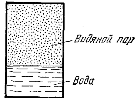
Рис. 1.38. Здесь показано совместное существование двух фаз, воды и пара, находящихся в равновесии при некоторой определенной температуре. Давление пара зависит только от температуры.
