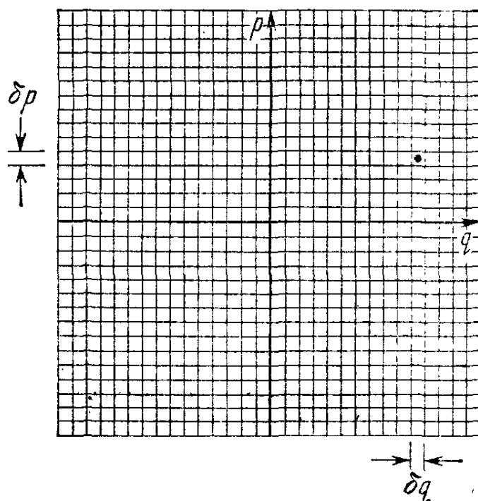
Рис. 6.2. Двумерное фазовое пространство предыдущего рисунка разделено на ячейки равного «объема» \delta q \delta p = h_0 .
