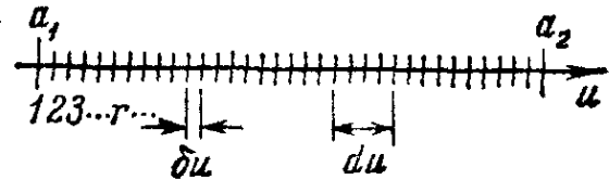
Рис. 2.13 Область изменения непрерывной переменной u разделена на счетное число малых интервалов одинакового размера \delta u . Каждый такой интервал обозначен индексом, принимающим значения 1, 2, 3, ... На графике показана также величина макроскопически малого интервала du .
