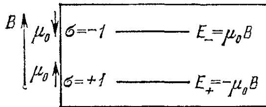
Рис. 3.2. На диаграмме показаны два уровня энергии, принадлежащие спину 1/2 , имеющему магнитный момент \mu_0 и находящемуся в магнитном поле \mathbf{B} . Состояние, помеченное \sigma = +1 (или просто + ) отвечает магнитному моменту, направленному вверх, т. е. по магнитному полю \mathbf{B} . Состояние \sigma = -1 (или - ) соответствует направлению магнитного момента вниз.
