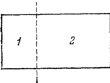
Рис. 5.15. Разделение однородной макроскопической системы на две части
