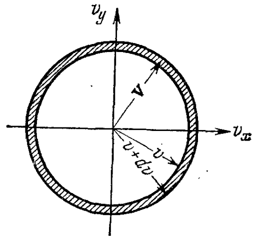
Рис. 6.6. Пространство скоростей для двух измерений (ось v_z перпендикулярна к плоскости чертежа). Сферический слой содержит все молекулы, скорость которых \mathbf{v} такова, что v < |\mathbf{v}| < v + dv .
