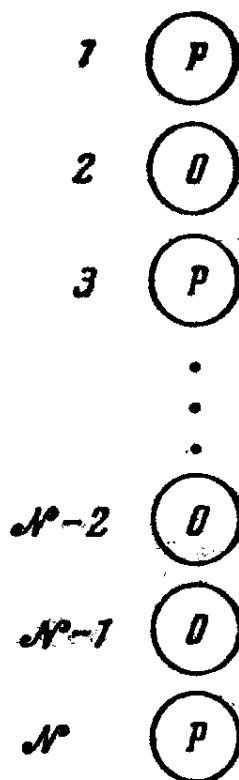
Рис. 2.1. Чтобы сделать предсказания о вероятных результатах бросания данной монеты, рассмотрим ансамбль, состоящий из большого числа одинаковых монет. На рисунке показано состояние ансамбля после бросания всех монет. Символ O означает «орел», символ P — «решка».
