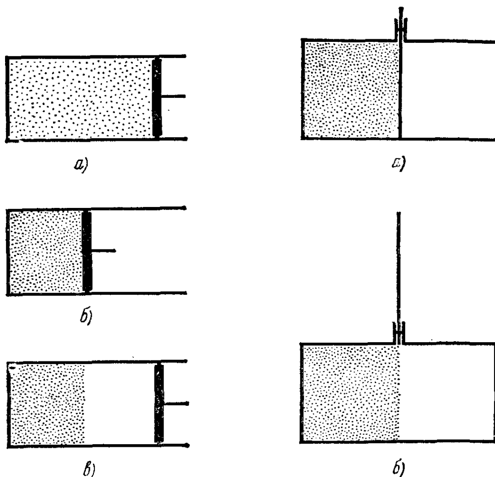
Рис. 1.10. Когда перегородка (a) неожиданно убирается, все молекулы в первый момент остаются в левой половине сосуда (б).
