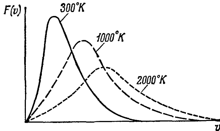
Рис. 6.8. Максвелловское распределение скоростей молекул при различных температурах.
