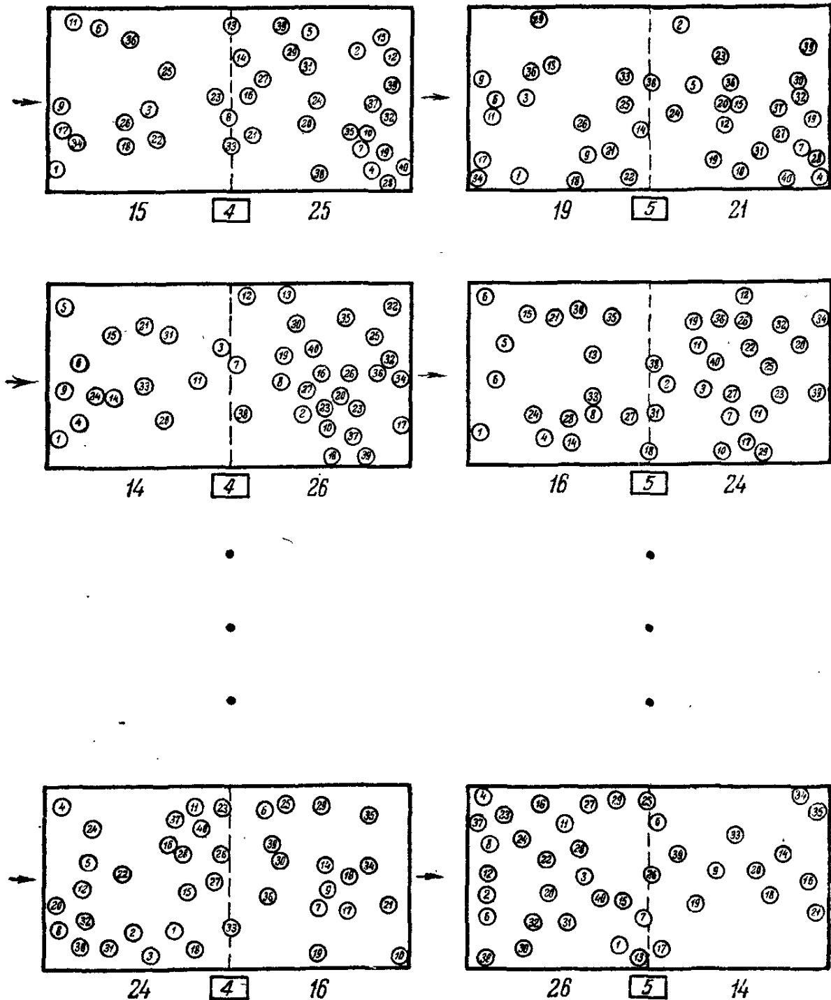
Рис. 2.4. Продолжение рис. 2.3. Теперь, когда прошло достаточно время, ансамбль является независимым от времени. Это означает, что система достигла состояния равновесия.
