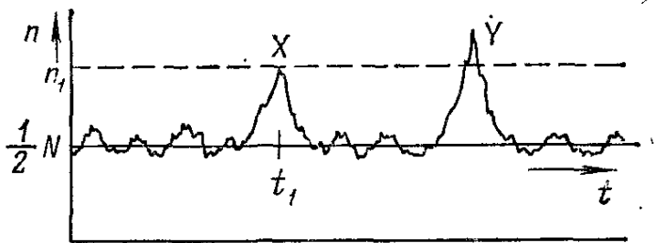
Рис. 1.8. Диаграмма, показывающая редко возникающие большие флуктуации числа молекул n в одной половине сосуда относительно равновесного значения 1/2 N .
