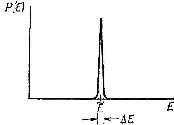
Рис. 4.2. Характер зависимости вероятности P(E) от энергии E .
